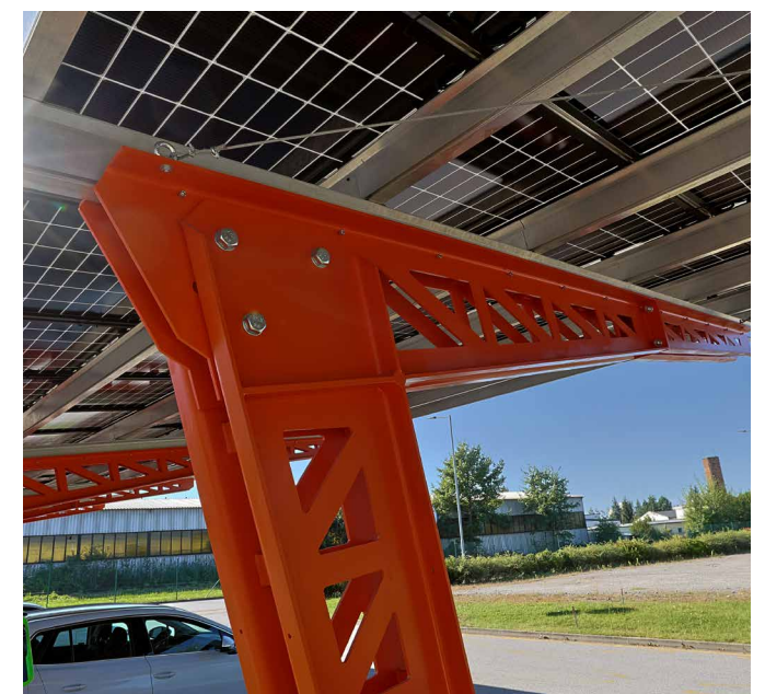
Detail kloubového uložení
